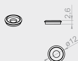
PPK-PODKŁADKA PCV
