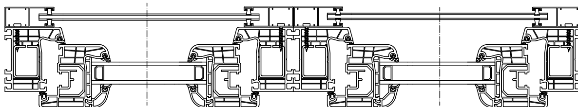
Montaż prowadnic prostych PP-53 oraz prowadnicy podwójnej PPD-79 - typ montażu B.
