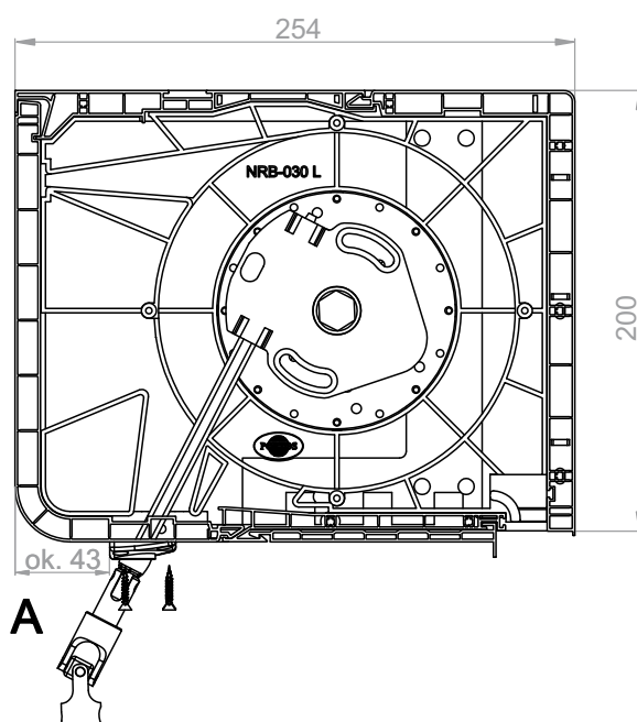
Skrzynka 200 Korbowy mechanizm podnoszenia z przegubem kardana Wyjście A od dołu przy pokrywie bez uchwytu
