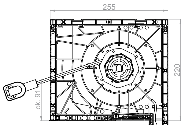
Skrzynka 220 Silnik z awaryjnym ręcznym podnoszeniem (NHK) Wyjście od czoła.
