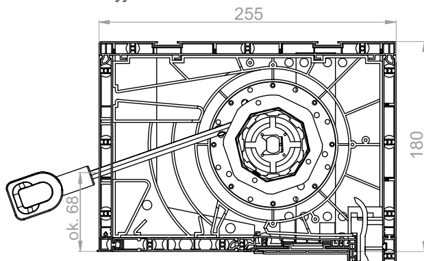
Skrzynka 180 Silnik z awaryjnym ręcznym podnoszeniem (NHK) Wyjście od czoła.
