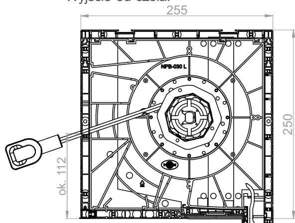
Skrzynka 250 Silnik z awaryjnym ręcznym podnoszeniem (NHK) Wyjście od czoła.
