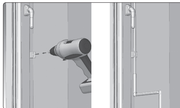
21. W rolecie z napędem ręcznym przykręcić zwijacz do ramy.
