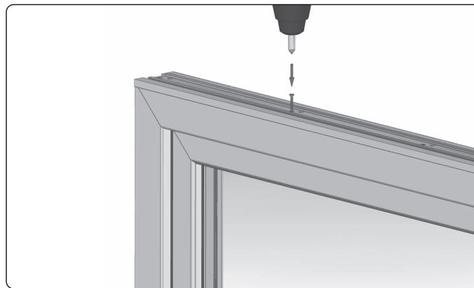
3. W odległości 10 cm od brzegu przykręcić zamontowane części adaptera. W razie potrzeby przewiercić otwór wiertłem 3 mm, a następnie nafrezować wiertłem 8 mm.
