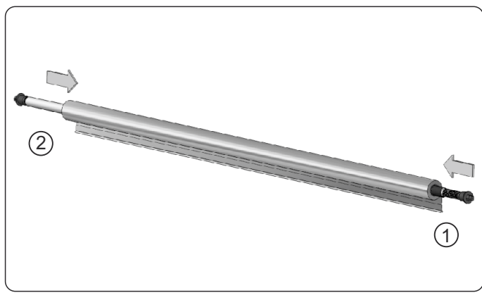
7. Die Bremse (1) und die Feder (2) in die Insektenschutz-Welle stecken. Achten Sie darauf, dass die Nase an der Feder der Bremse in die Öffnungen in der Insektenschutzwelle einrastet.
