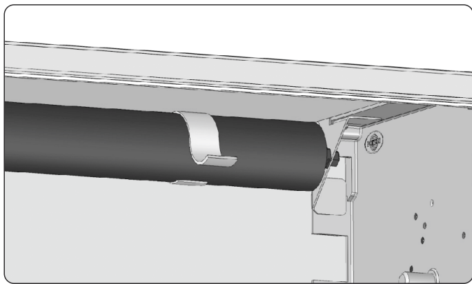
13. Das Insektenschutzgitter festhalten und die Abrollssicherung (Papierband) abnehmen.
