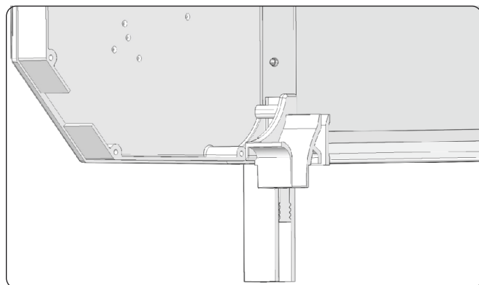
2. Den oberen Teil des Kastens vernieten.
