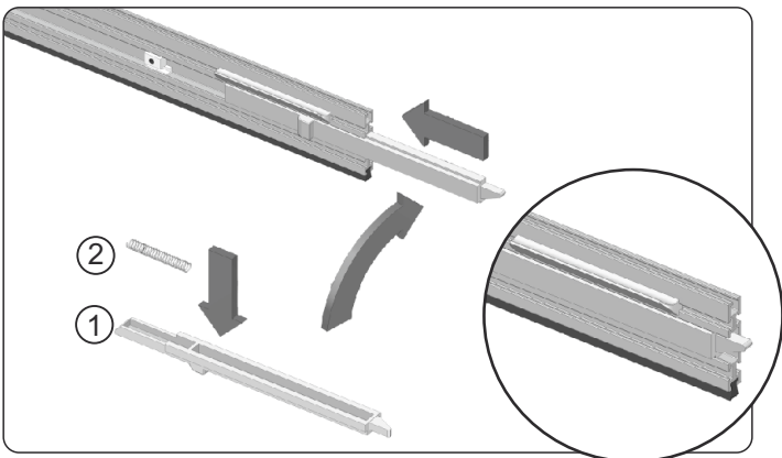
6. Die Feder (2) in das untere Teil des Riegels (1) stecken, das Ganze in den Kanal der Insektenschutz-Endschiene, in dem sich die Riegelsperre befindet, einschieben. Den Riegel mit der Feder auf die Sperre drücken.
