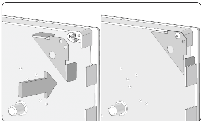
1. Den Insektenschutzhalter an die Blendkappe halten und montieren.
