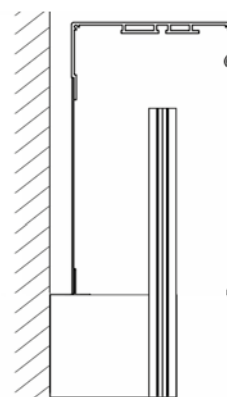
TYP D - Skrzynka na elewację z odsadzeniem. Dedykowane przewody F-FBR-020.
