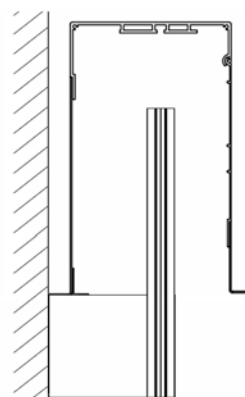
TYP B - Skrzynka pod zabudowę z odsadzeniem. Dedykowane prowadnice F-FBR-040.
