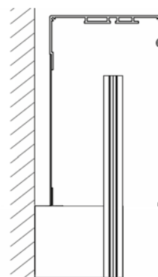
TYP D - Skrzynka na elewację z osadzeniem. Dedykowane prowadnice F-FBR-020.
