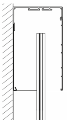
TYP C - Skrzynka na elewację. Dedykowane prowadnice F-FBR-010.
